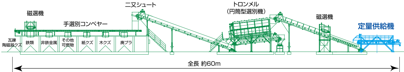
側面図
