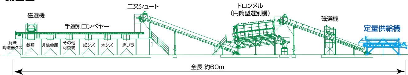
側面図
